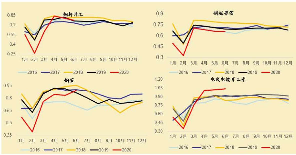
图 2：铜材开工率
