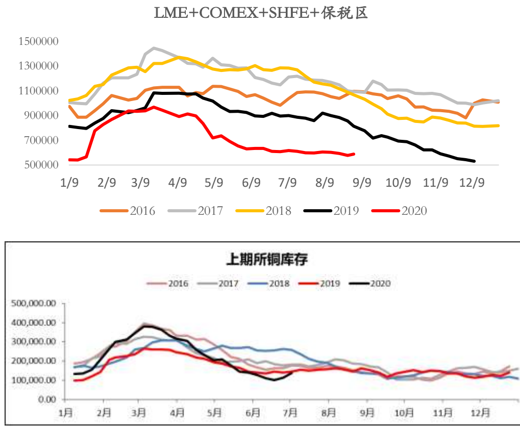
图 4：铜库存
